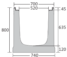
Hoogte 800
