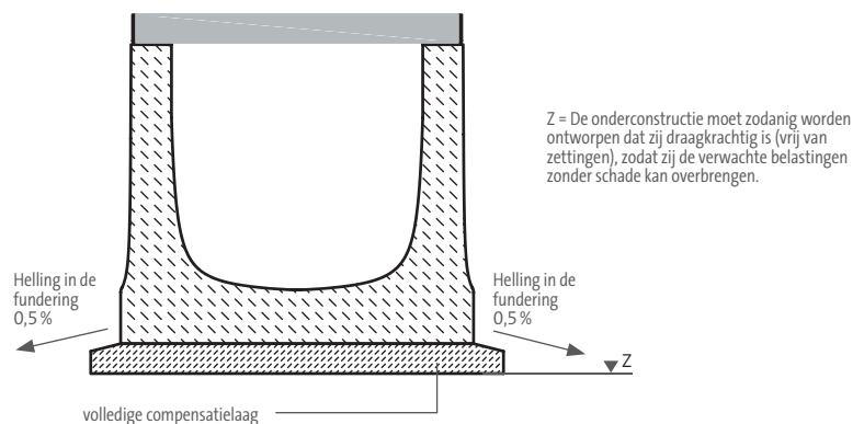
Afbeelding met goottype BIRCOsir®
