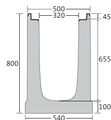
Hoogte 800
