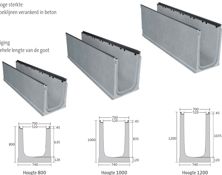
Hoogte 800
