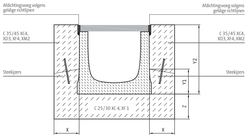
Afbeelding met goottype BIRCOsir®
