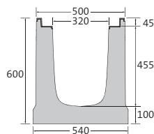
Hoogte 600
