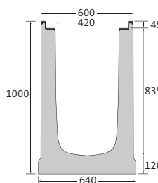
Hoogte 1000
