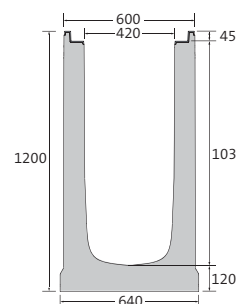
Hoogte 1200
