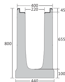
Hoogte 800
