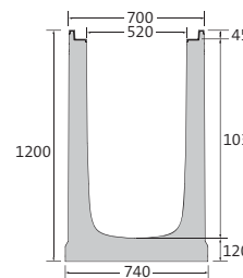
Hoogte 1200
