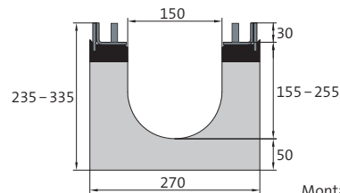
Montagevoorbeeld
