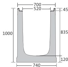
Hoogte 1000
