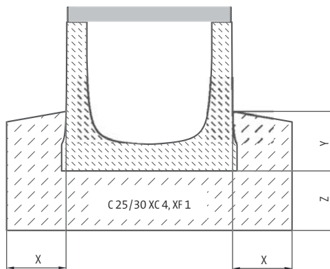
Afbeelding met goottype BIRCOsir®
