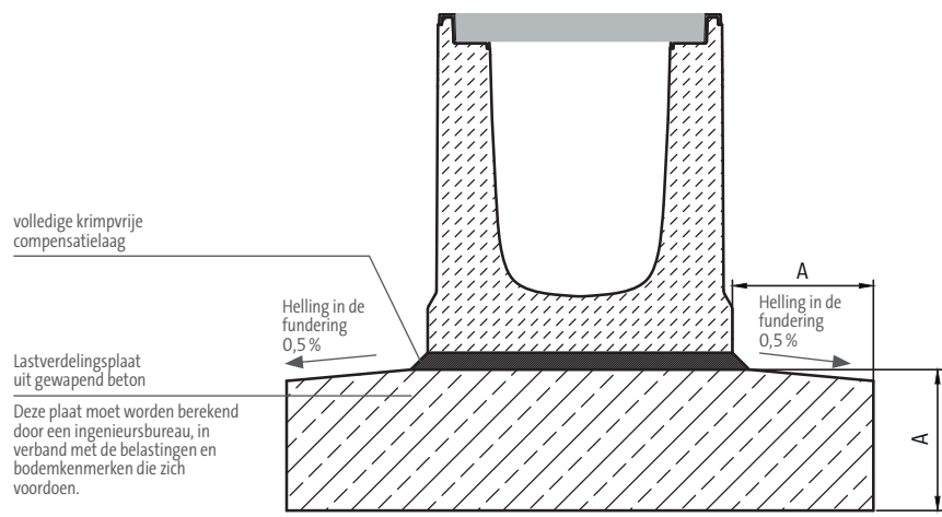
Afbeelding met goottype BIRCOmax-i®
