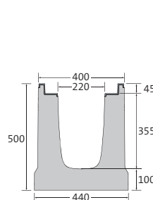
Hoogte 500
