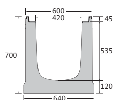
Hoogte 700
