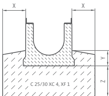
Afbeelding met goottype BIRCOsir®
