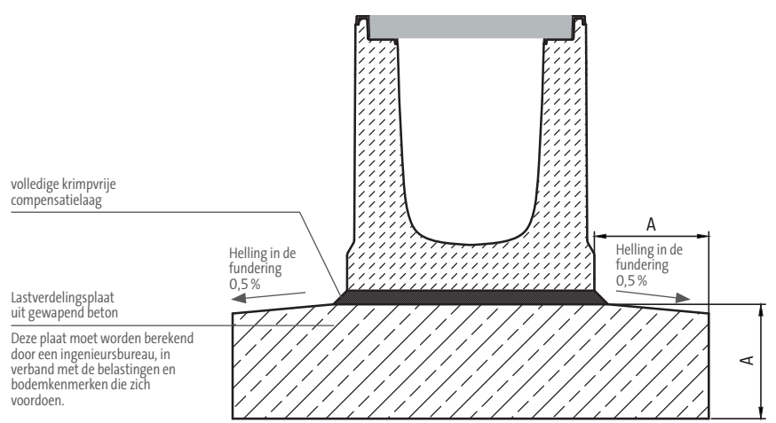
Afbeelding met goottype BIRCOmax-i®
