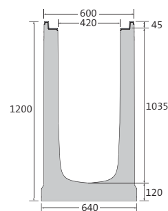
Hoogte 1200
