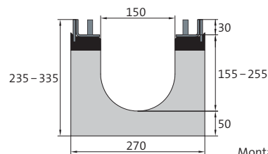
Montagevoorbeeld
