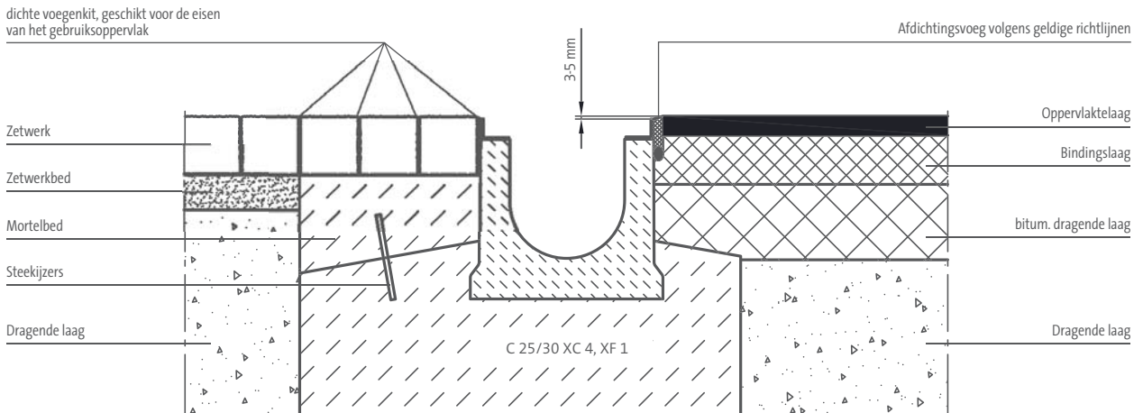
Aanleg van vorstbestendige draag- en funderingslagen (vrije samenstelling) overeenkomstig: "Catalogus van standaardwegconstructies" / "Richtlijnen voor grondwerken bij wegenbouw" Een verdichtingsvrije ondergrond die is afgestemd op de gebruiksbelastingen.
