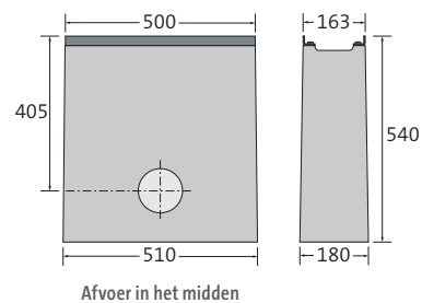
Afvoer in het midden
