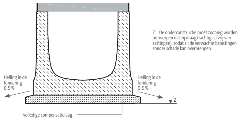
Afbeelding met goottype BIRCOsir®
