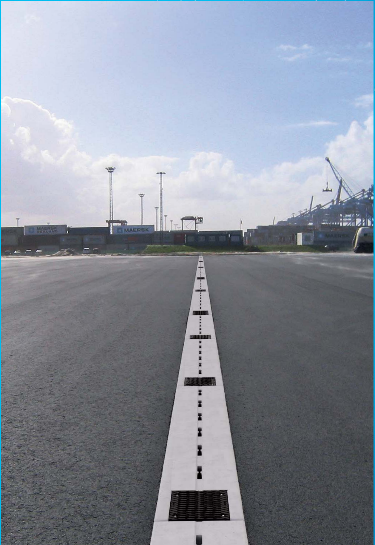
BIRCOsolid® Sleufgoot voor de afwatering van een haveninstallatie
