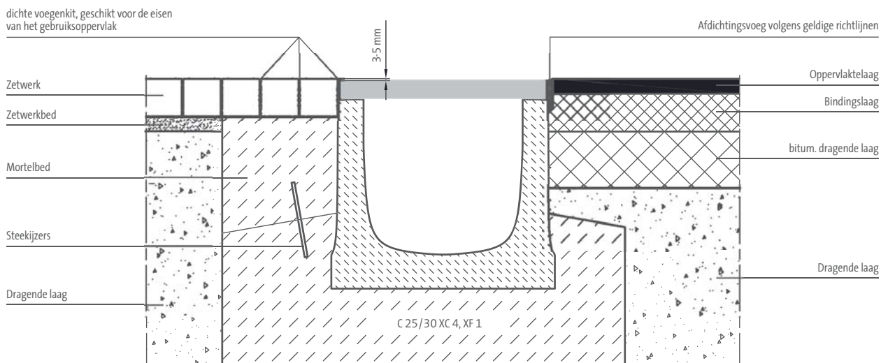
Aanleg van vorstbestendige draag- en funderingslagen (vrije samenstelling) overeenkomstig: "Catalogus van standaardwegconstructies" / "Richtlijnen voor grondwerken bij wegenbouw" Een verdichtingsvrije ondergrond die is afgestemd op de gebruiksbelastingen.
