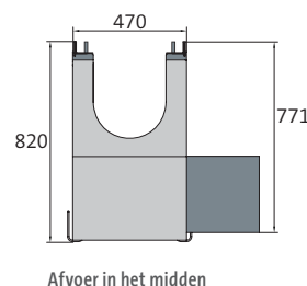
Afvoer in het midden
