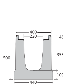
Hoogte 500
