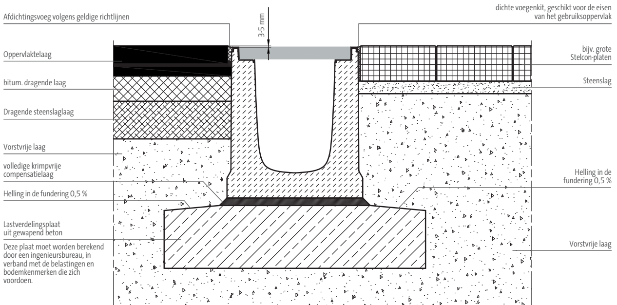
Aanleg van vorstbestendige draag- en funderingslagen (vrije samenstelling) overeenkomstig: "Catalogus van standaardwegconstructies" / "Richtlijnen voor grondwerken bij wegenbouw" Een verdichtingsvrije ondergrond die is afgestemd op de gebruiksbelastingen.
