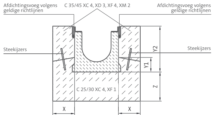
Afbeelding met goottype BIRCOsir®
