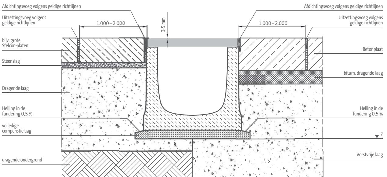
Aanleg van vorstbestendige drag- en funderingslagen (vrije samenstelling) overeenkomstig: "Catalogus van standaardwegconstructies" / "Richtlijnen voor grondwerken bij wegenbouw" Een verdichtingsvrije ondergrond die is afgestemd op de gebruiksbelastingen.
