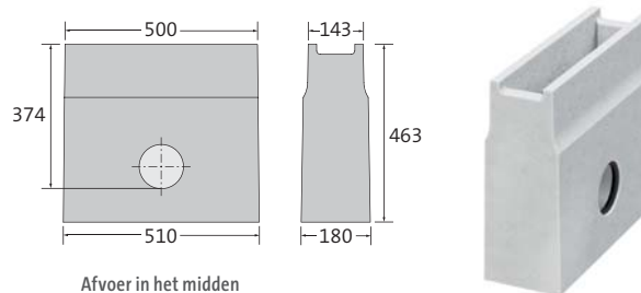
Afvoer in het midden
