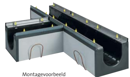
Montagevoorbeeld
