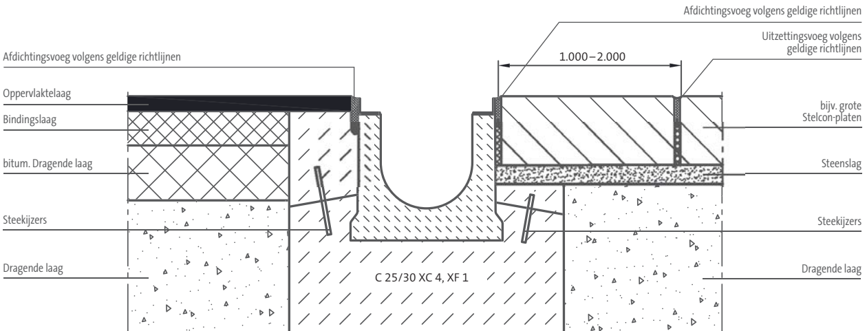
Aanleg van vorstbestendige draag- en funderingslagen (vrije samenstelling) overeenkomstig: "Catalogus van standaardwegconstructies" / "Richtlijnen voor grondwerken bij wegenbouw" Een verdichtingsvrije ondergrond die is afgestemd op de gebruiksbelastingen.
