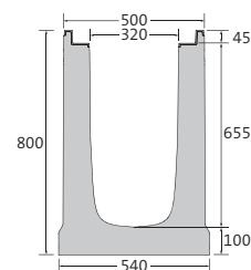
Hoogte 800
