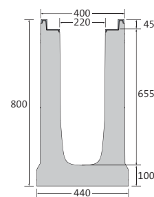
Hoogte 800
